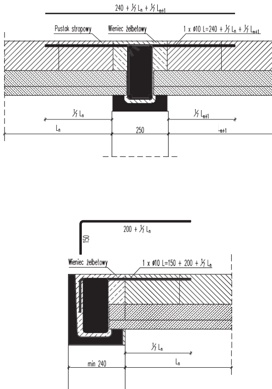
Rys. 1 Zbrojenie nadpodporowe.
